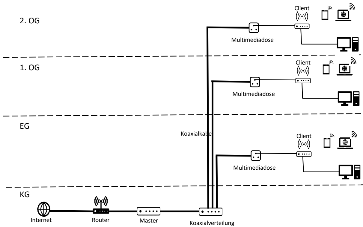
Abbildung 14: Koaxialnetzwerk
